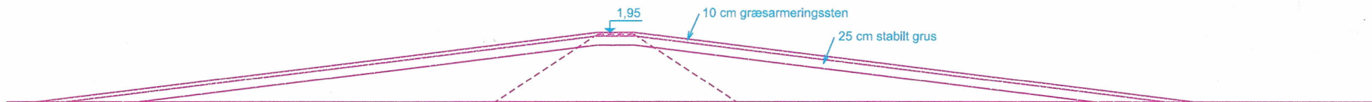
Principielt tværsnit i overkørsel
