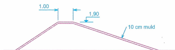
Principielt tværsnit i dige
